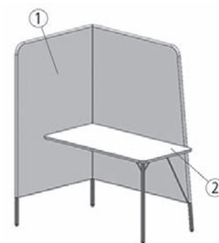
m.zone single levý – pracovní výška 740 mm složený z: ① 1 zástěna ② 1 pracovní deska Bez ilustrace: m.zone single pravý – pracovní výška 740 mm
