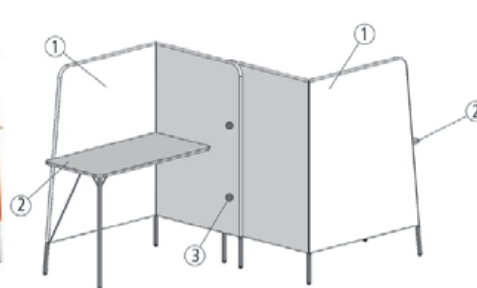
m.zone double – pracovní výška 900 mm složený z: ① 2 zástěny ② 2 pracovní desky ③ 2 spojovače
