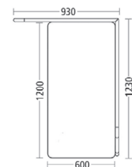
m.zone single levý – pracovní výška 740 mm složený z: ① 1 zástěna ② 1 pracovní deska Bez ilustrace: m.zone single pravý – pracovní výška 740 mm
