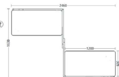
m.zone double – pracovní výška 900 mm složený z: ① 2 zástěny ② 2 pracovní desky ③ 2 spojovače
