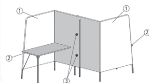
m.zone double – pracovní výška 740 mm složený z: ① 2 zástěny ② 2 pracovní desky ③ 2 spojovače
