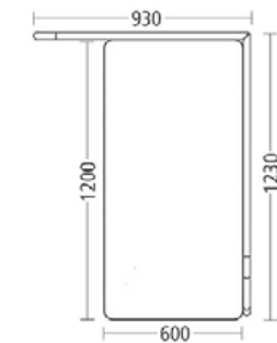
m.zone single levý – pracovní výška 900 mm složený z: ① 1 zástěna ② 1 pracovní deska Bez ilustrace: m.zone single pravý – pracovní výška 900 mm
