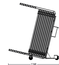
Uskladňovací vozík 6398-000 (příklad při délce stolu 1600)
